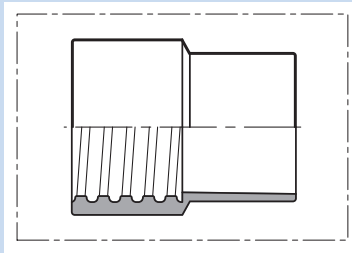
miękką złączka do węży z EVA
